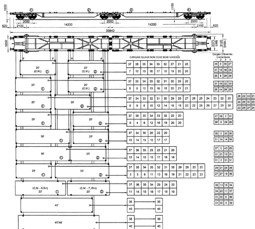
Diagrama de cargas
